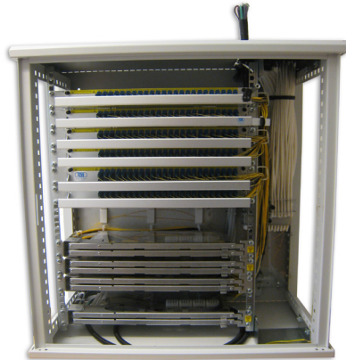
Termineringsbox T596
